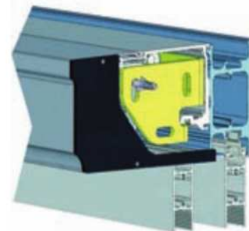
Cajón entre pared: Escuadras de fijación/Tapas laterales troqueladas
